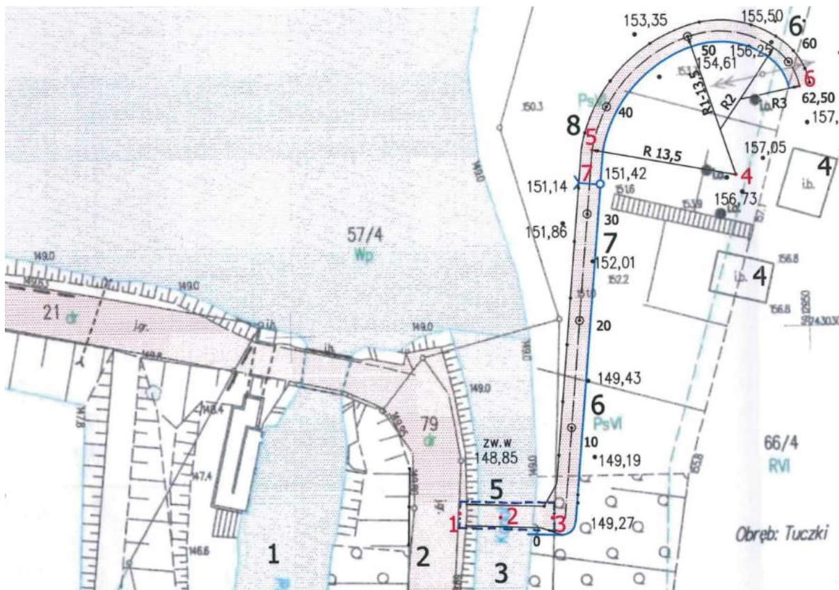
Dokumentacja budowy kładki na rzece Wel
